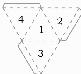
नियमित त्रिभुजाधार पिरामिड
