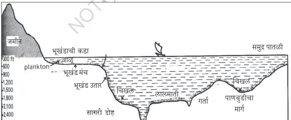
महासागरचा तळ
